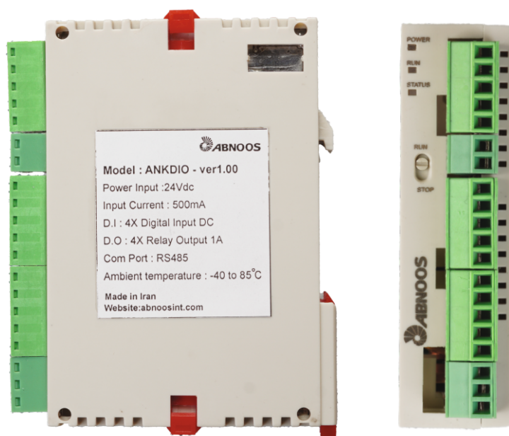
Modbus Digital I/O Module
